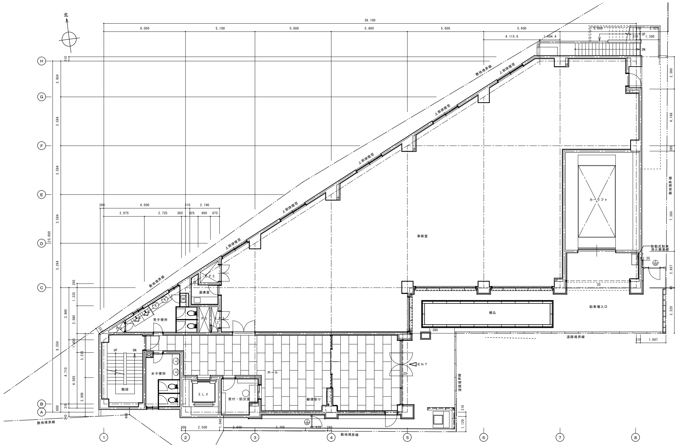
1階平面図 S = 1 / 60
